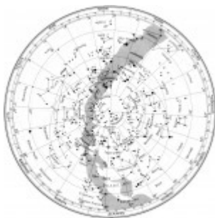
Подвижная карта звездного неба
